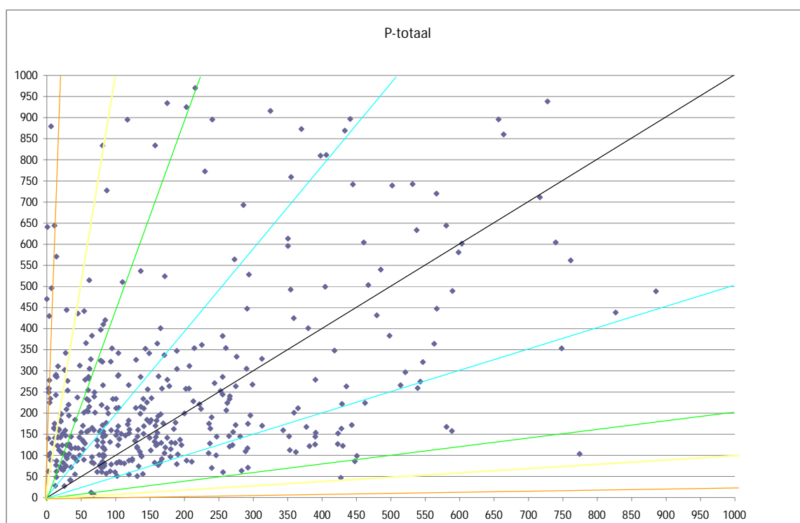
Figuur 5.3 Relatiediagram van de berekende jaargemiddelde concentraties (X-as) uitgezet tegen de gemeten jaargemiddelde concentraties (Y-as). De zwarte lijn is de "ideale lijn". Punten tussen de blauwe lijnen wijken maximaal een factor 2 af van de "ideale lijn" en punten tussen de groene lijnen maximaal een factor 5. Binnen de gele lijnen maximaal een factor 10 en binnen de oranje lijnen maximaal een factor 50.
